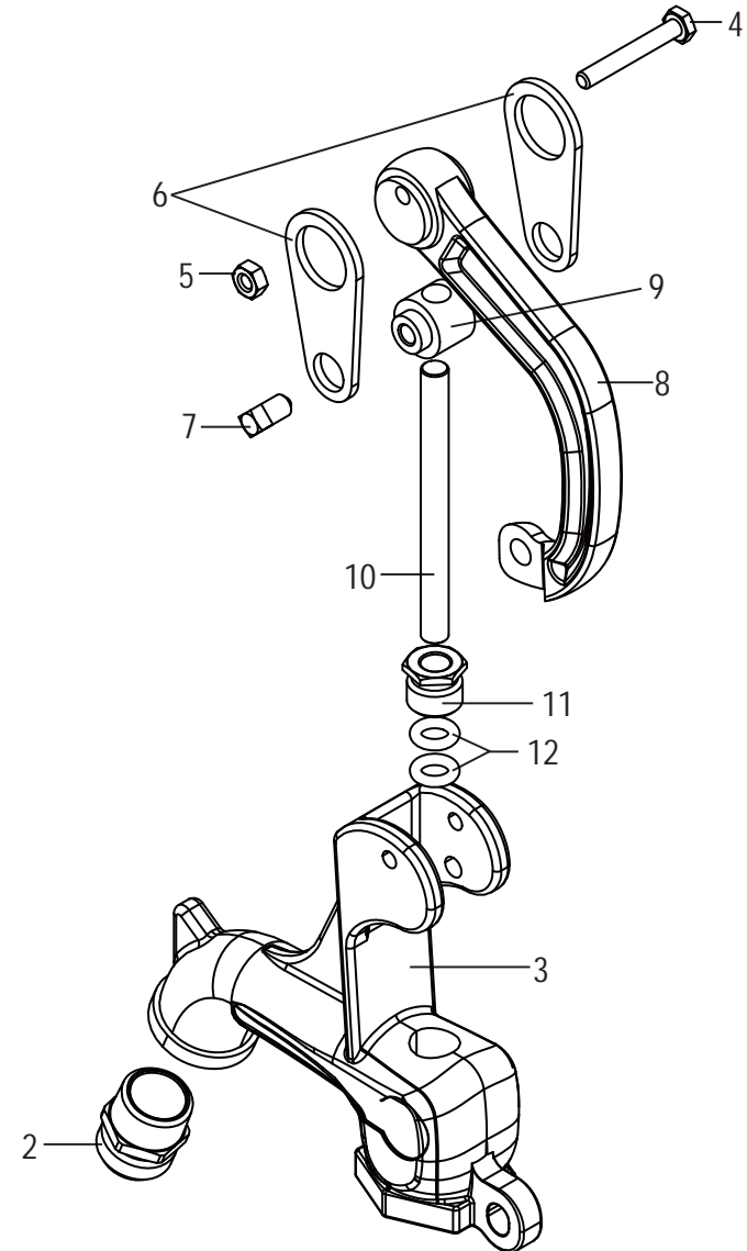
YHC-RED & YHHD-RED Exploded View
